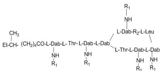
图 1 多黏菌素的化学结构式
